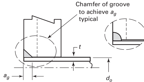
Groove Weld (b)
