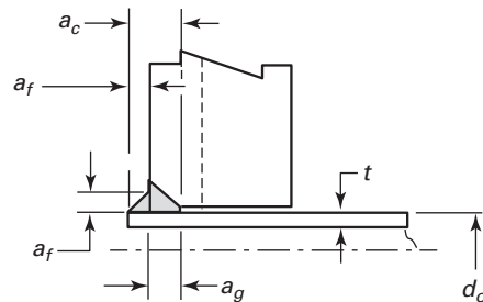
Combination Face-Fillet and Groove where: a_c = a_f + a_g and a_f \neq a_g (d)
